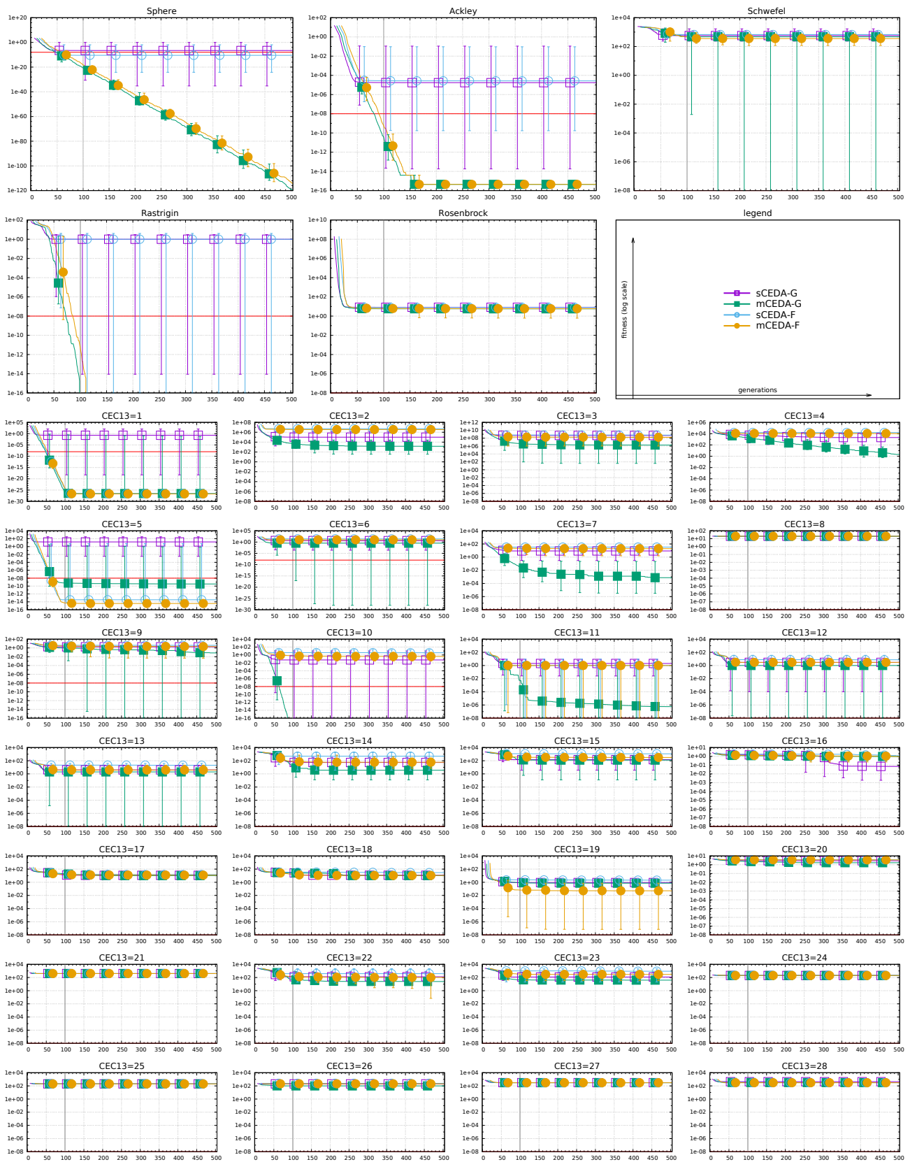
Obrázek 1. Výsledky experimentů – medián a kvartily hodnoty fitness algoritmů s Gaussovou a Frankovou kopulí; sekvenční verze a verze s migrací modelů.
